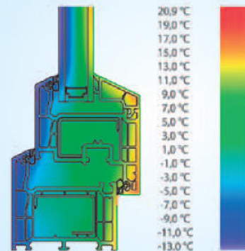
Průběh izoterm
