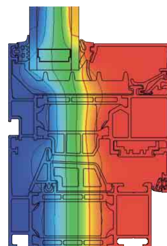
Der neue Wärmedämmstandard für Aluminium-Fenster AWS 75.SI The new thermal insulation standard for aluminium windows AWS 75.SI
