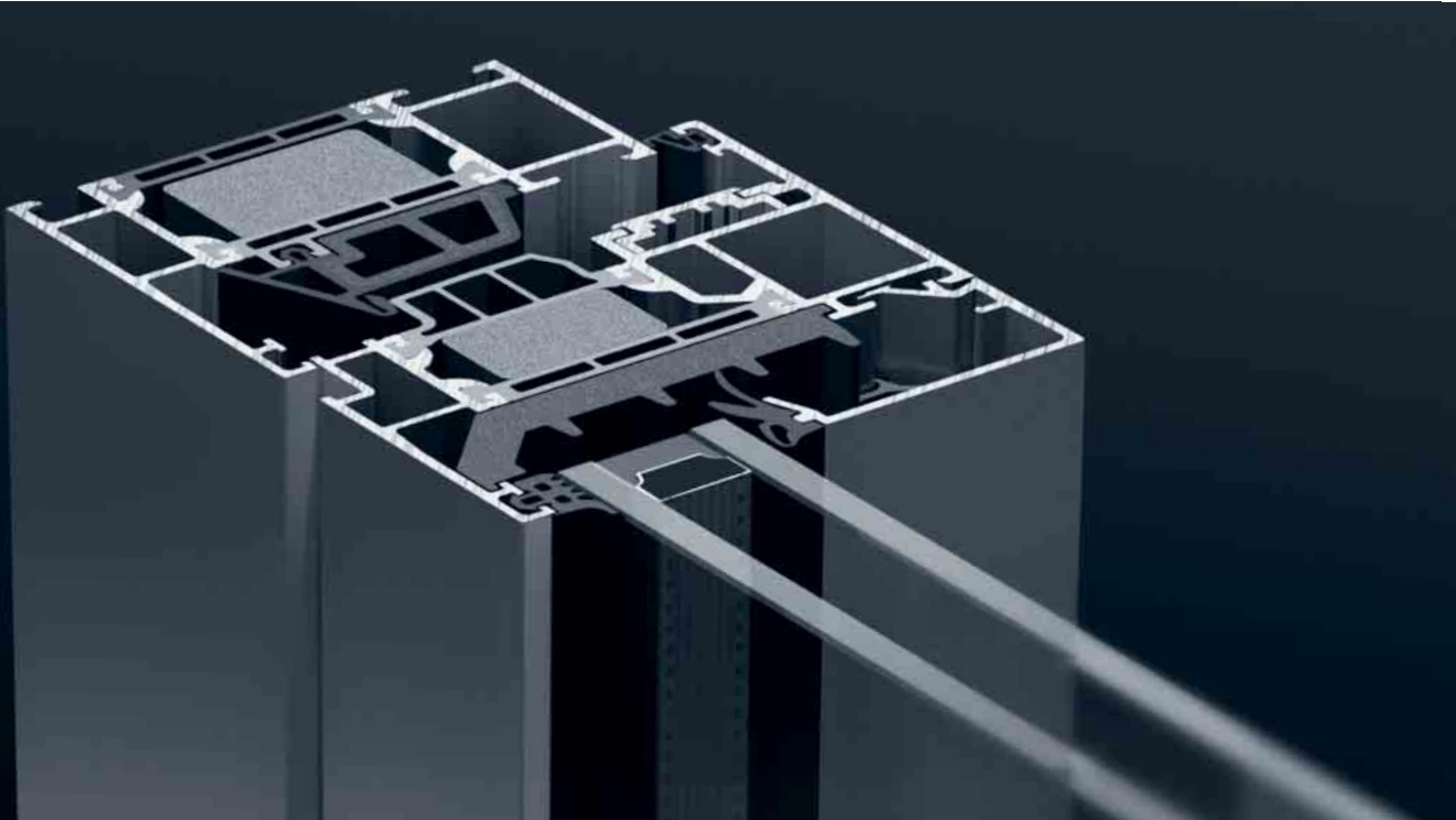
Schüco AWS 75.SI: Höchster Wärmedämmwert ( U_f 1,4 W/m 2 K), Ansichtsbreite von 117 mm Schüco AWS 75.SI: the highest thermal insulation value ( U_f 1.4 W/m 2 K) with a face width of 117 mm
